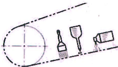
Figura 14: Método de lubrificação de correntes.
