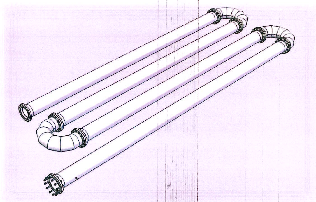
Figura 5: Representação tubulação de reação físico-química.
