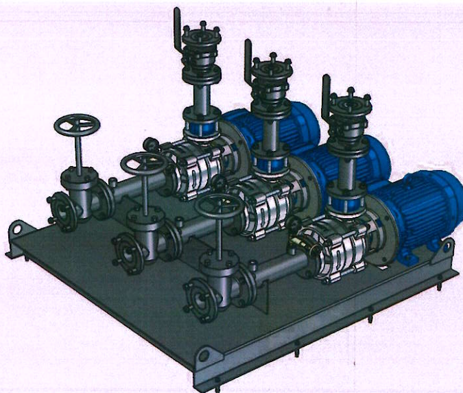
Figura 7: Representação sistema de recirculação triplo.
