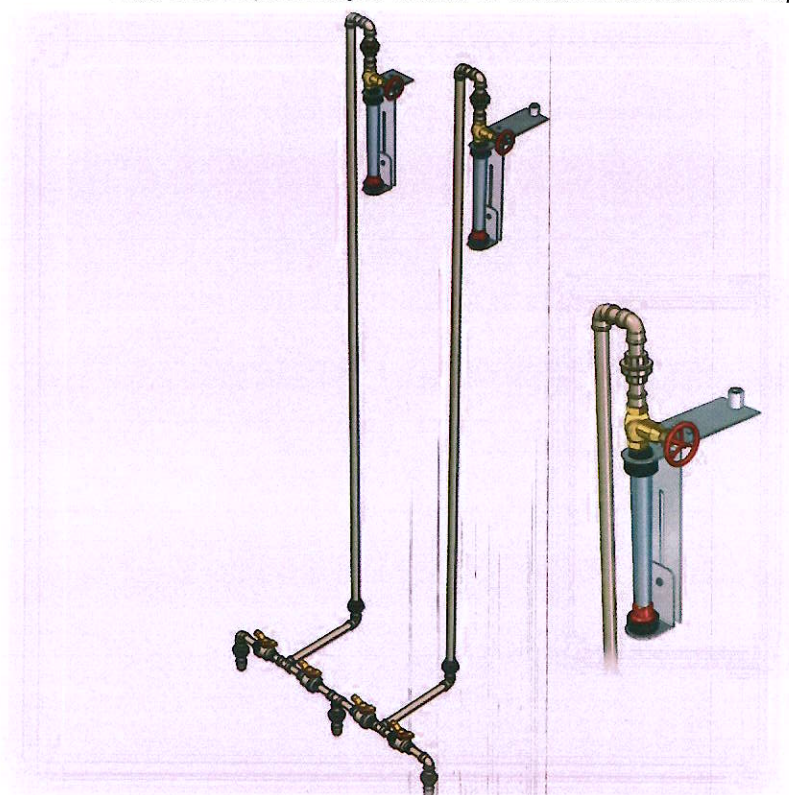
Figura 11: Representação sistema de entrada e controle de ar duplo.
