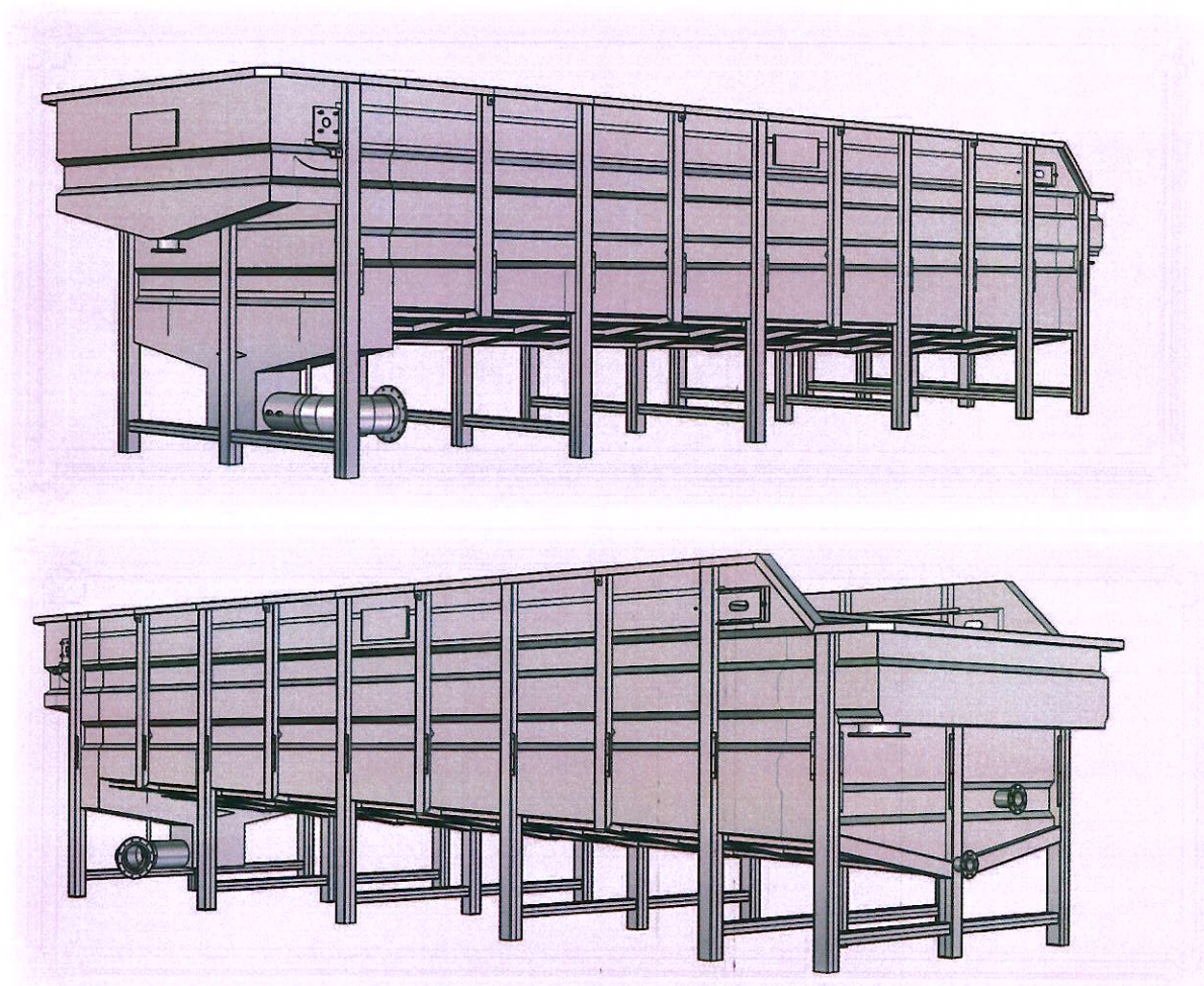
Figura 4: Tanque de flotação GFAD 300I.
