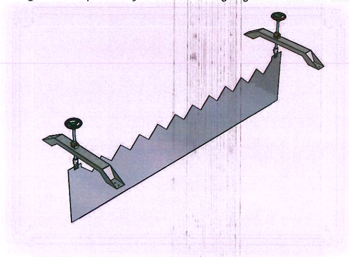
Figura 12: Representação sistema de regulagem da saída do clarificado.
