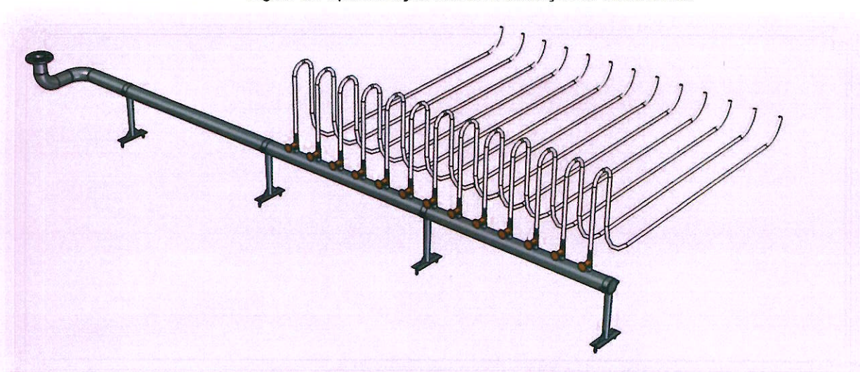
Figura 9: Representação tubo de distribuição de microbolhas.
