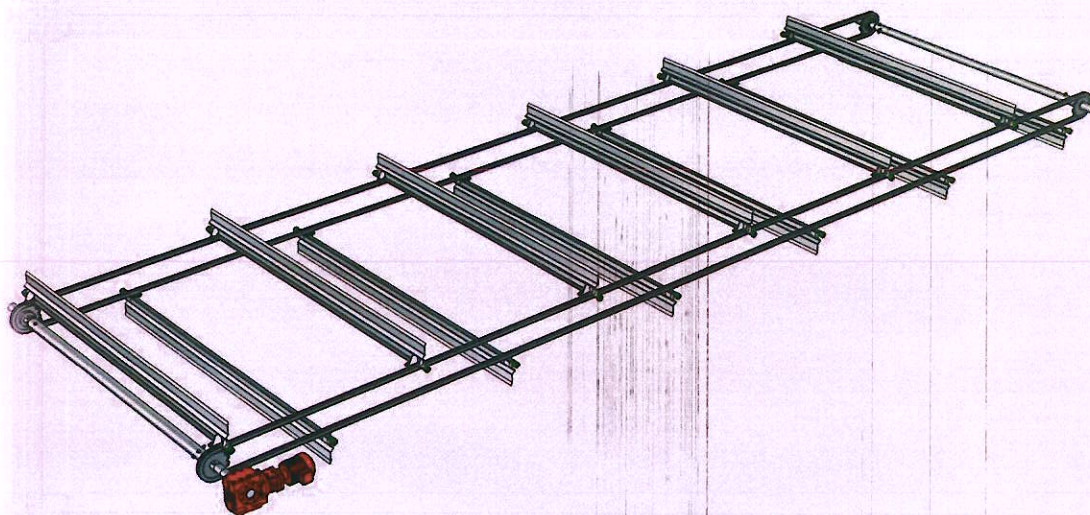
Figura 6: Representação sistema de raspagem de lodo flotado.
