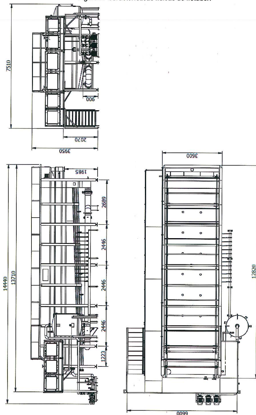
Figura 2: Características físicas do flotor.
