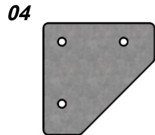
04 P03150021 x4 Chapa Reforço Tubos ITR-1200 (Z)
