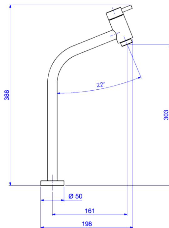
Desenho Técnico
